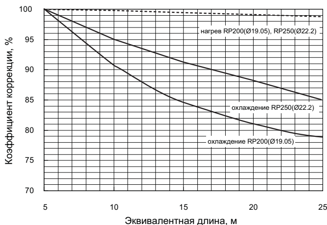
3) График 3. Диаметр газовой трубы на 2 типоразмера меньше стандартного значения.
