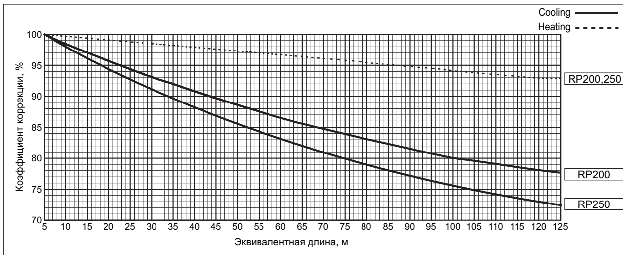
1) График 1. Диаметр газовой трубы имеет стандартный типоразмер.
