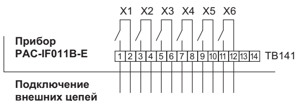
Рис. 3. Подключение внешних цепей к прибору PAC-IF011B-E.
